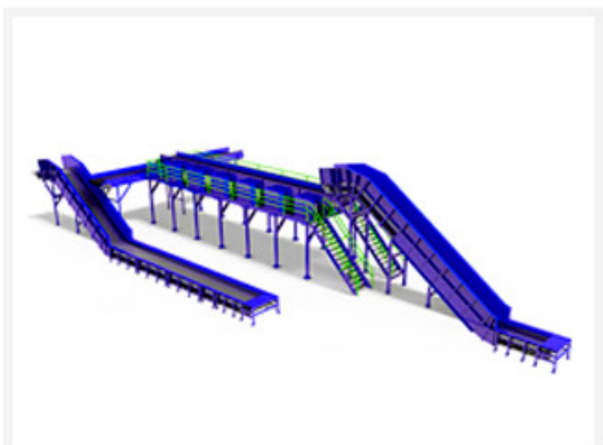
Автоматическая сортировка ТБО
